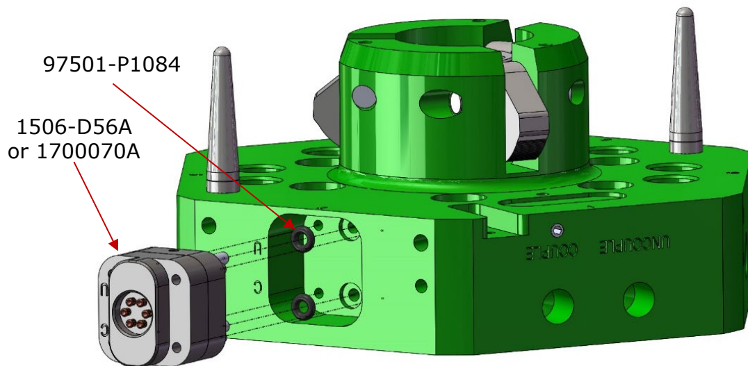
Figure 10.1.2-1. Couple/Uncouple Sensing Module Replacement
