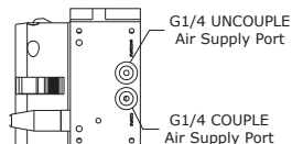
VIEW A-A
