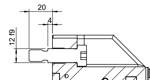
SEZIONE C-C
