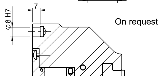
SEZIONE A-A
