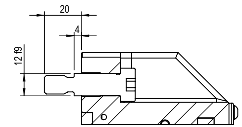
SEZIONE K-K
