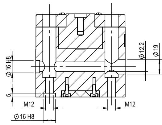
SEZIONE B-B
