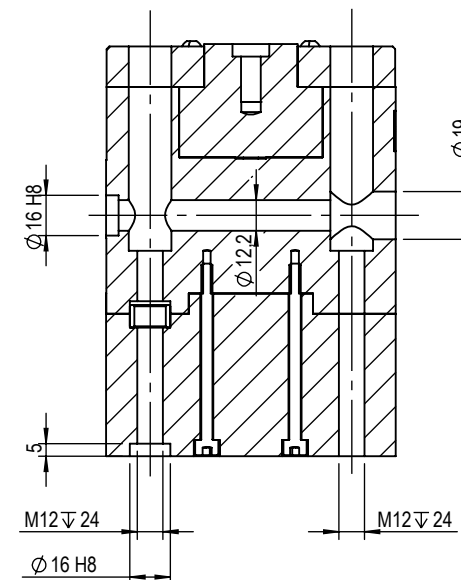
SEZIONE B-B
