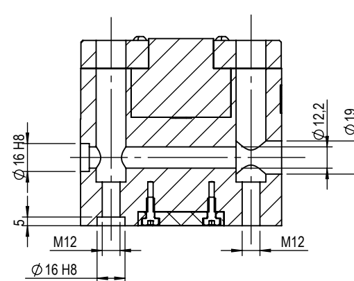
SEZIONE B-B
