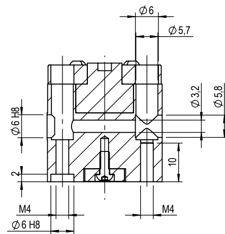
SEZIONE A-A SCALA 1 : 1
