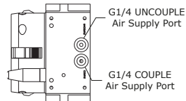
VIEW A-A
